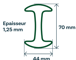
Section du poteau
