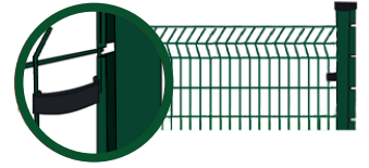
4. Installer les cales d'écartement pour fixer le panneau pendant le séchage du béton.
